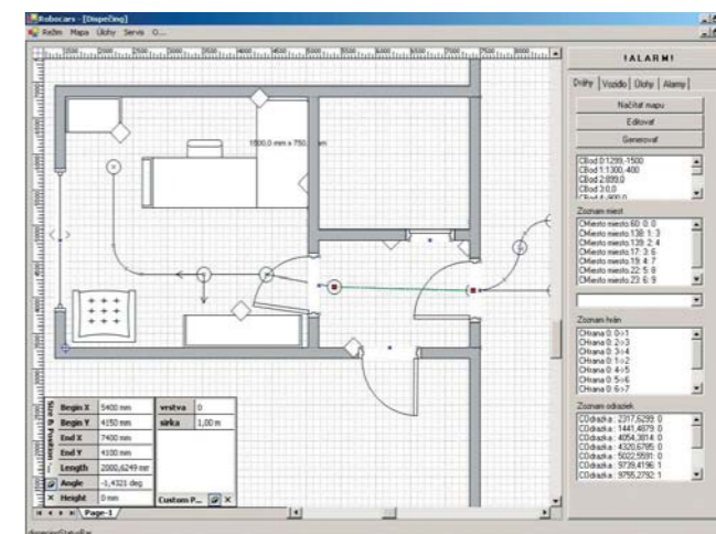
Obr.4 Příklad dráhového systému
