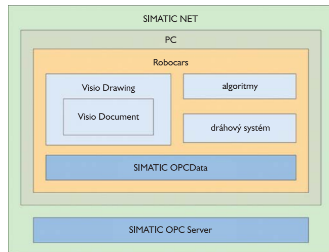
Obr.1 Štruktúra softvéru
